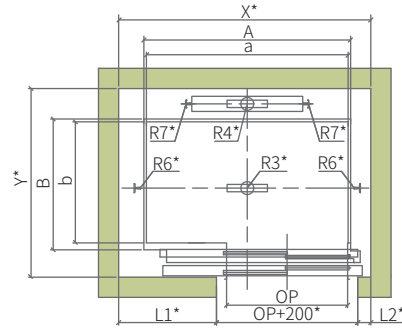
井道平面图 (开门形式: 2P-CO, 偏心门)
