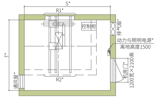
井道平面图 (开门形式: 2S-2P, 左开门)
