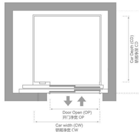
单通门 Single door
