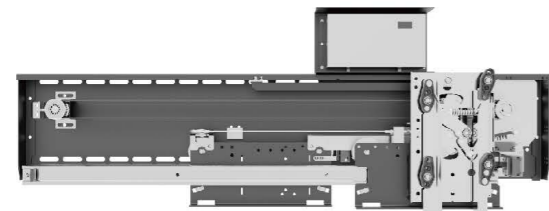
PMA2S-Z 双折式门机装置 Side open door operator
